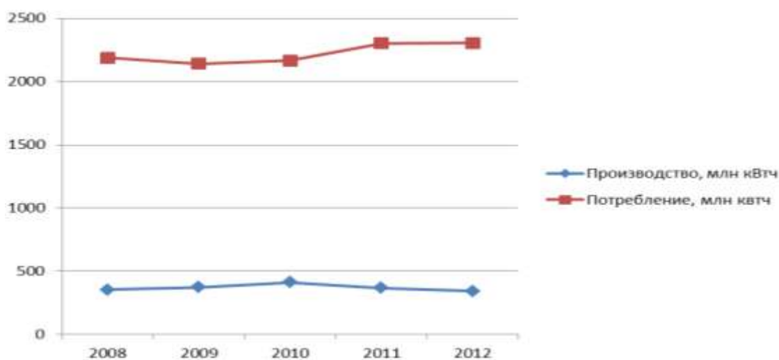
Динамика потребления и производства электроэнергии в Республике Северная Осетия-Алания за последние 5 лет (по данным системного оператора)
